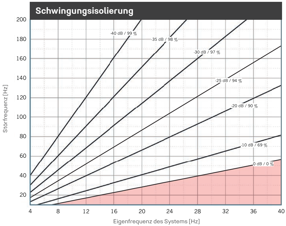
Dargestellt ist die Isolierung für einen Ein-Massen-Schwinger auf starrem Untergrund mit REGUPOL vibration 800 . Parameter: Kraftübertragungsmaß in dB, Isolierwirkungsgrad in %.
